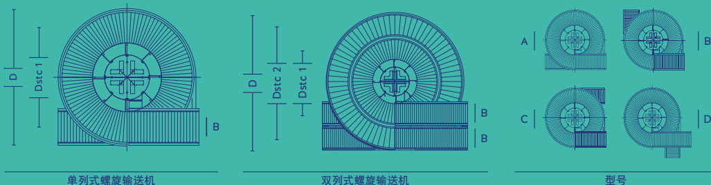
单列式螺旋输送机
